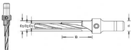
vrták na confirmáty - stavitelný
